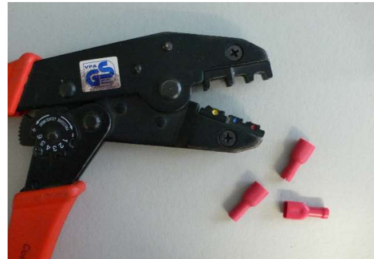
Crimpzange und Flachsteckhülsen
